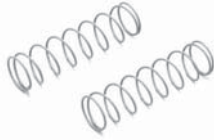
IS106-7514 *1100 ビッグダンパースプリング (M/グレー/7.5-1.4/L=84) Big Shock Spring (M/Gray/7.5-1.4/L=84)
