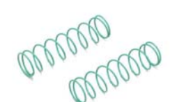
IS106-914 *1100 ビッグダンパースプリング (M/グリーン/9-1.4/L=84) Big Shock Spring (M/Green/9-1.4/L=84)
