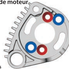
Positions du support de moteur
