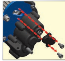
Extracción del cubierta del puerto para ver el engranaje
