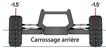
Carrossage avant
