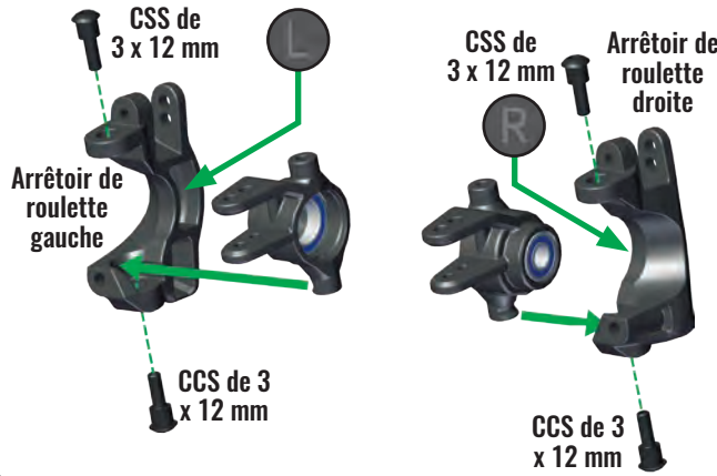
Assemblage de moyeu avant gauche
