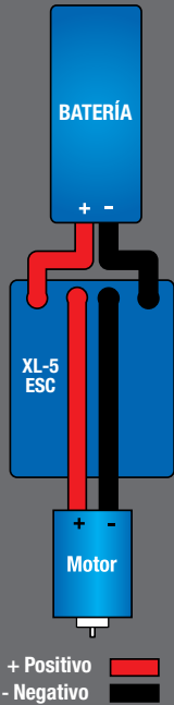
Diagrama de cableado del XL-5
